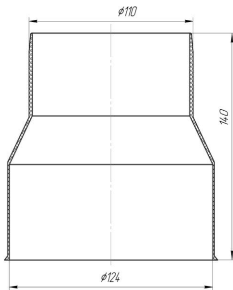
Переход ПП/ЧК 124/110
