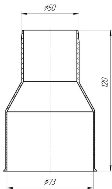
Переход ПП/ЧК 73/50
